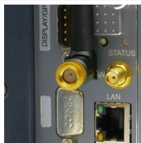
WLAN - Antenne mit SMA (männlich) Anschluss am Gerät SMA (weiblich)
