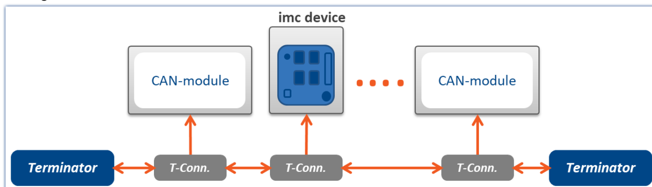
Messaerät mit angeschlossenem T-Stück
